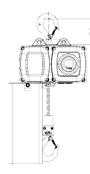
Model CPV/CPVF avec crochet de suspension, 250 - 2000 kg
