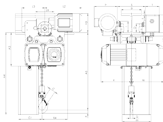
Modèle CPV/CPVF avec chariot électrique intégré
