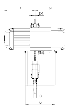
Modèle CPV/CPVF avec anneau de suspension, 500 - 5000 kg, 2 brins
